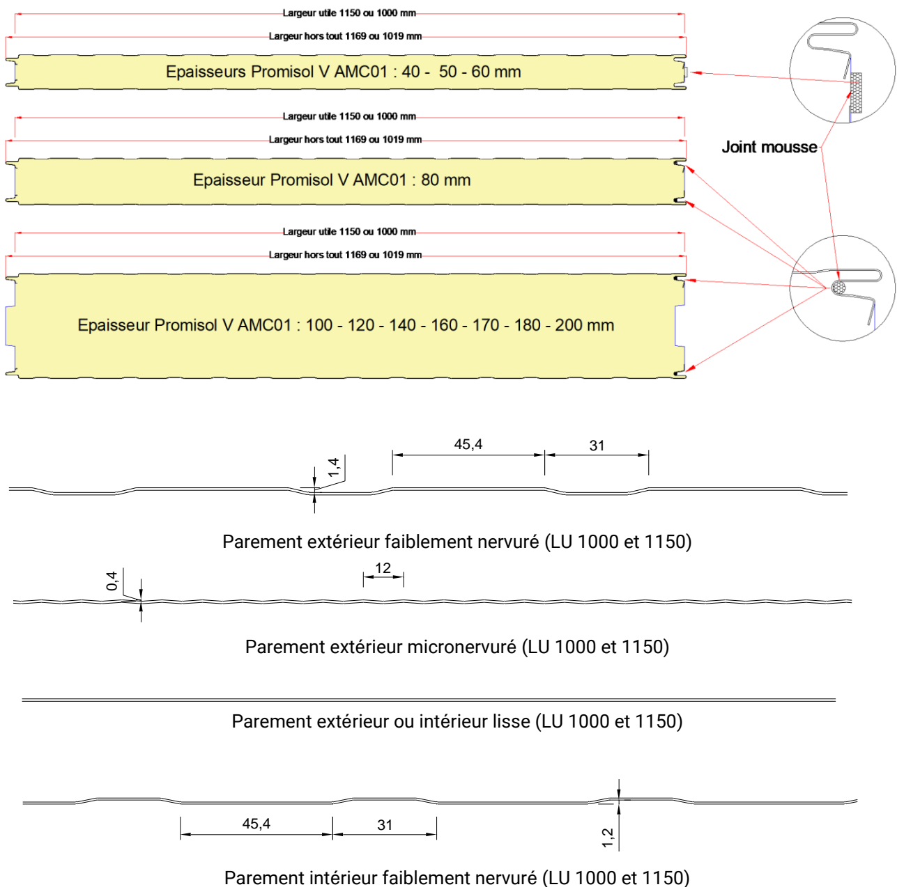
Figure 1 – Panneau Promisol V AMC 01 et ses parements (Toutes cotes en mm)
