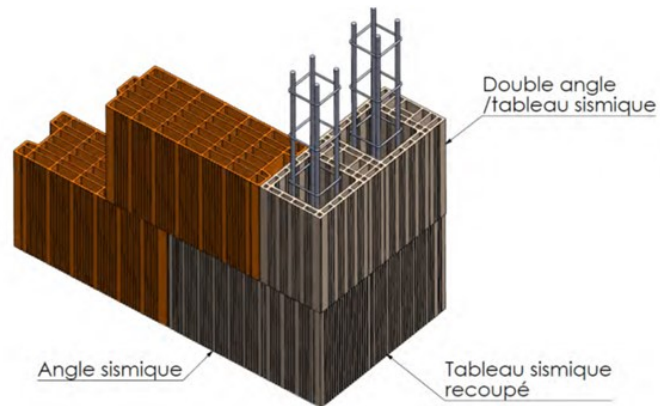
Liaison avec retour d'ouverture
