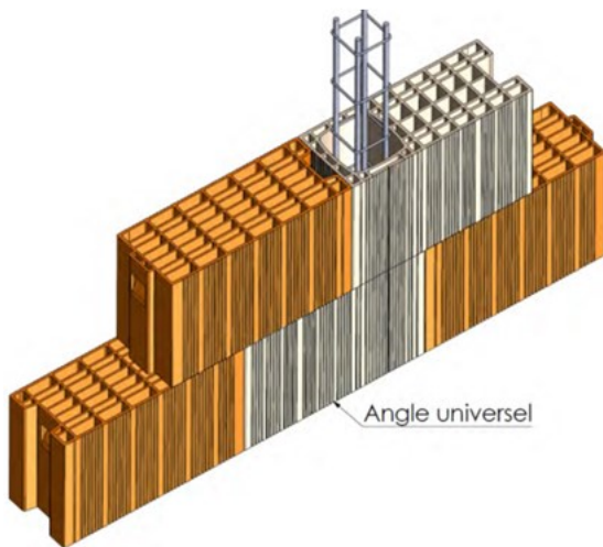
Poteau de contreventement
