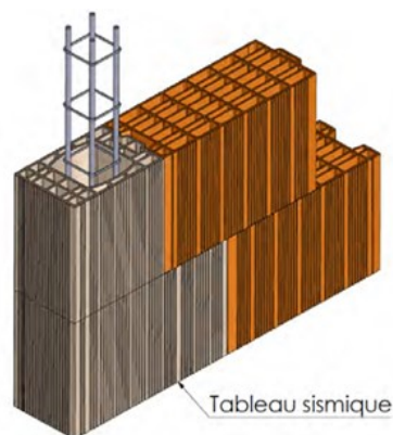
Liaison avec mur de refend
