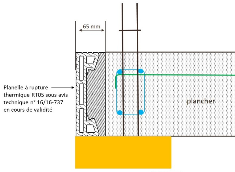
Coupes horizontales et verticales sur planelles à rupture thermique
