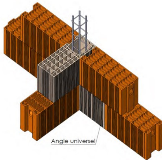
Liaison avec mur de refend
